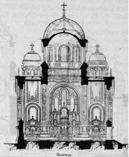
Чер. 328. Поперечный разръзъ.
