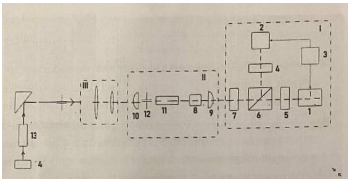
Рис.1.1 Функциональная схема инновационного стенда для сборки и юстировки лазерных излучателей с диодной накачкой.
