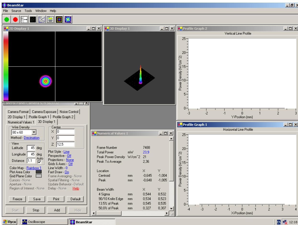
Рис.2 Профиль лазерного пучка в фокусе собирающей линзы с фокусным расстоянием 1 м
