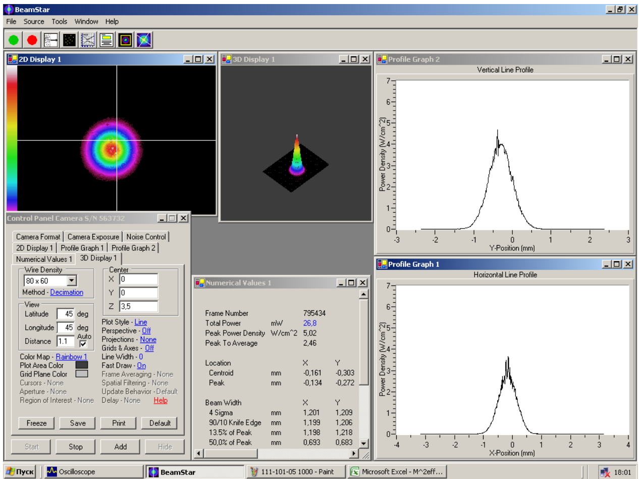
Рис.3 Профиль лазерного пучка на выходе лазера, полученная с применением ПЗС – камеры и компьютера.
