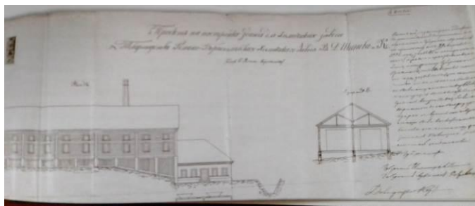
Фото 2. Проект постройки заводских зданий
